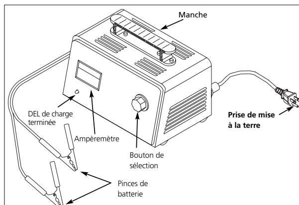
Figure 2 – Fonctions du chargeur de batterie Prise à la terre
